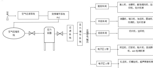
空氣壓縮管路圖
